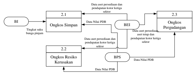
Gambar 7. DFD Level 2 (Ongkos Penanganan Persediaan)
