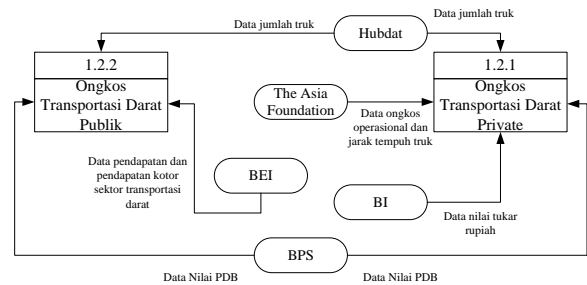
Gambar 8. DFD Level 3 (Ongkos Transportasi Darat)
